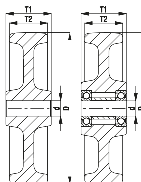
siklócsapágy golyócsapágy
